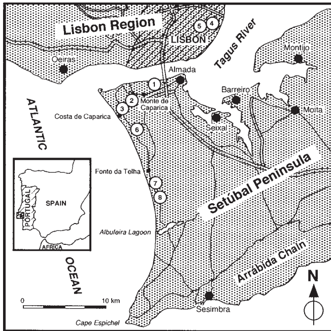
Figure 1. Geographic situation of odontocete localities within the distal part of the Lower Tagus Basin. 1. Palença de Baixo (SP). 2. Brielas (SP). 3. Costa de Caparica (SP). 4. Cerâmica Dias Coelho (LR). 5. Quinta do Alfundão (LR). 6. Foz do Rego (SP). 7. Fonte da Telha (SP). 8. Adiça (SP).
